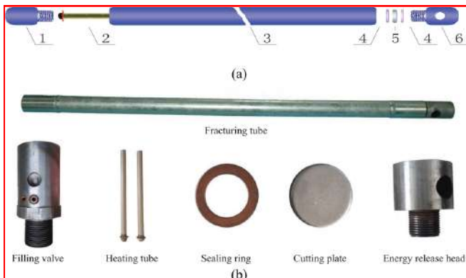
CARDOX CO2 BLASTING TUBE
